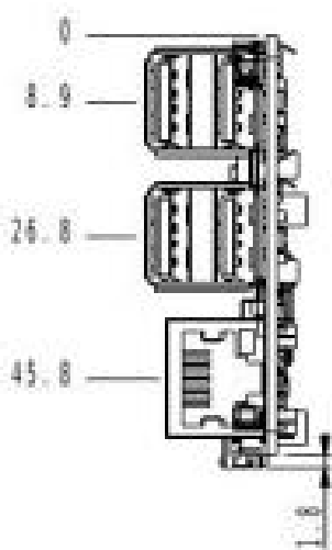
接口图
